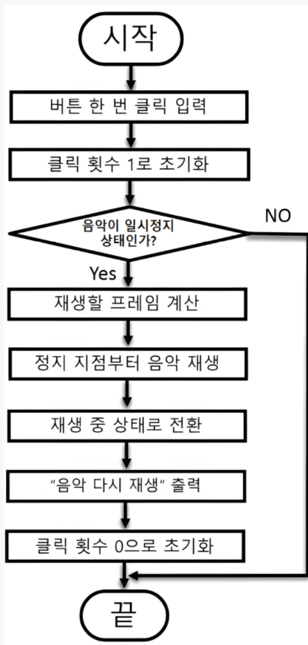
● 음악 다시 재생 순서도
