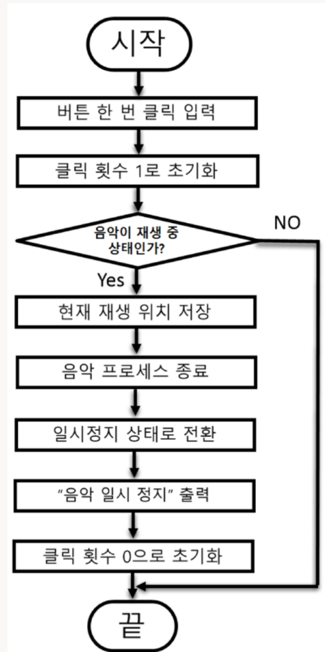
● 음악 일시정지 순서도
