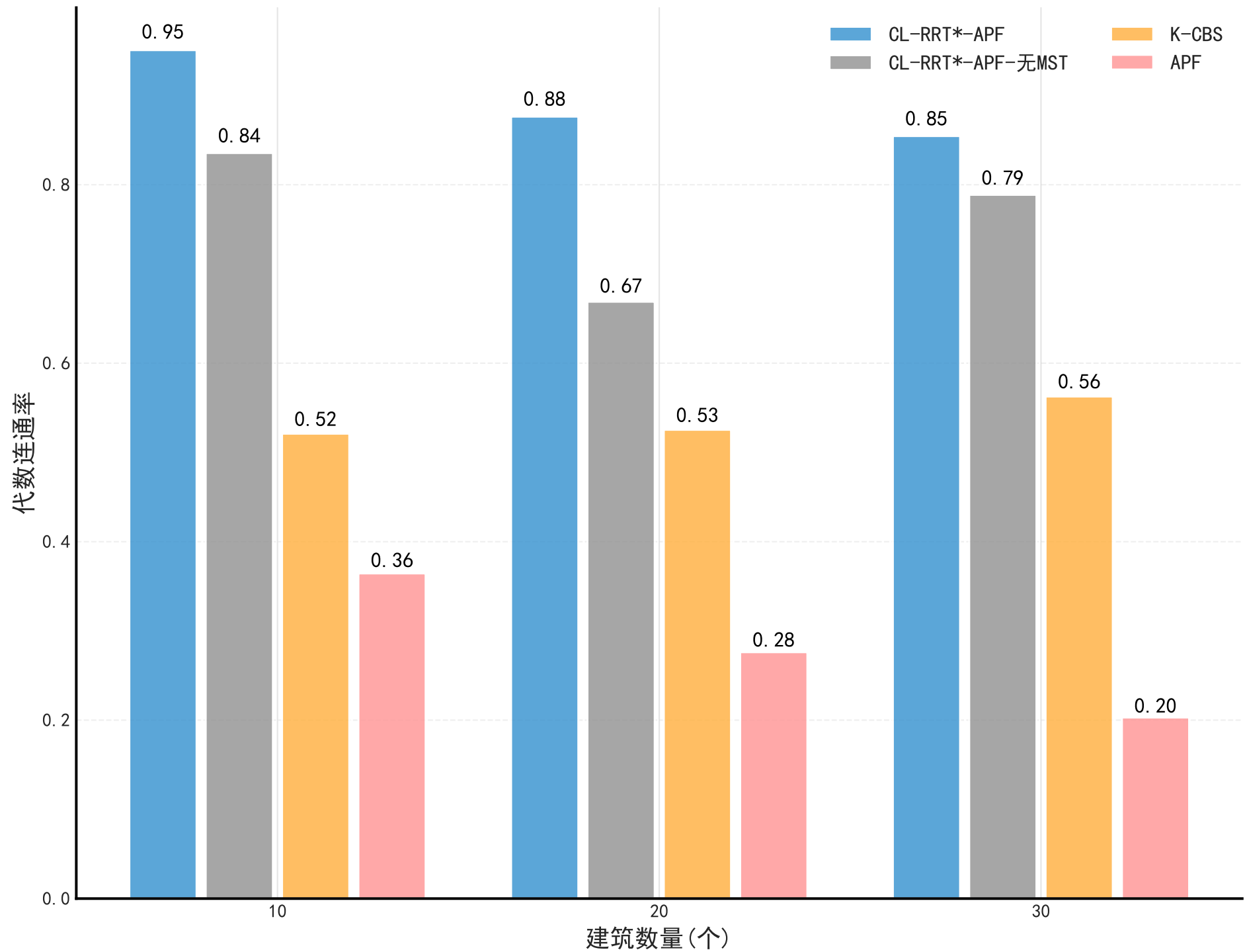
不同建筑数量下代数连通率对比结果
