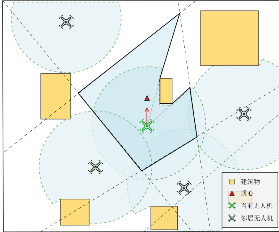
图4-3 Voronoi 覆盖引导算子原理示意图
