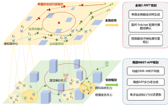
图2 C-RRT*-APF 算法框架示意图
