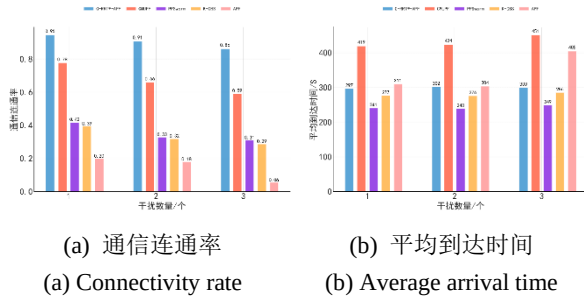
图5 不同干扰节点数量下的指标对比
