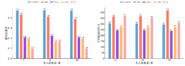
(a) 通信连通率 (b) 平均到达时间 (a) Connectivity rate (b) Average arrival time
