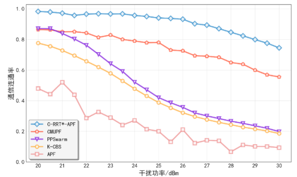
图6 通信连通率随干扰功率变化情况
