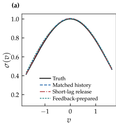
Brownian
