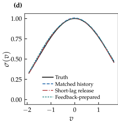
Brownian-Lévy
