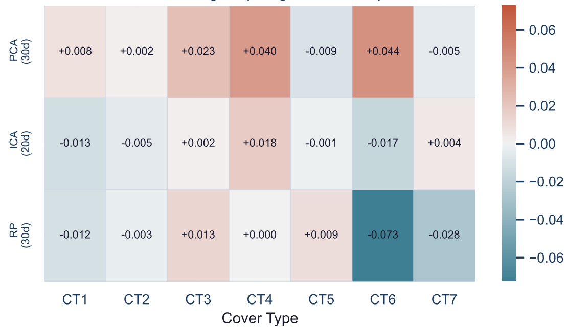
\Delta F1 vs. Original (red=gain, blue=loss)
