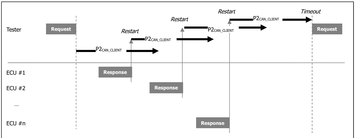
그림 2-8. P2 CAN_CLIENT timing parameter in Functional request
