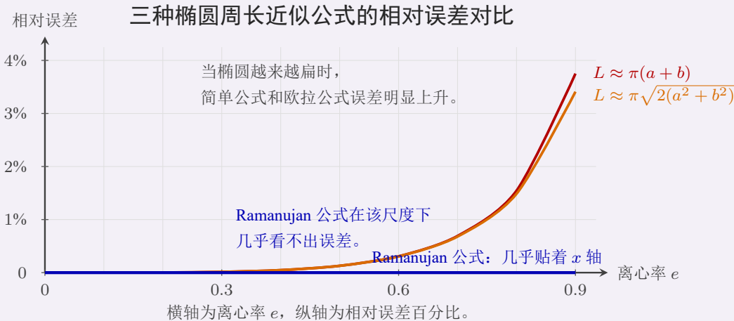
图：三种椭圆周长近似公式的相对误差对比
