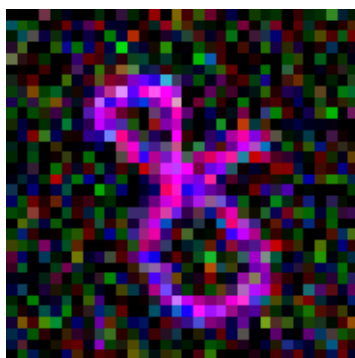
Huber ( \sigma=0.5 )
