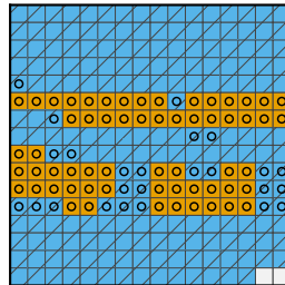
(d) ANATOMY-v2
