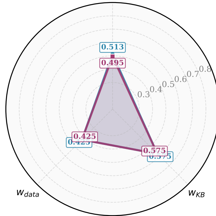
ECO Integrated F1
