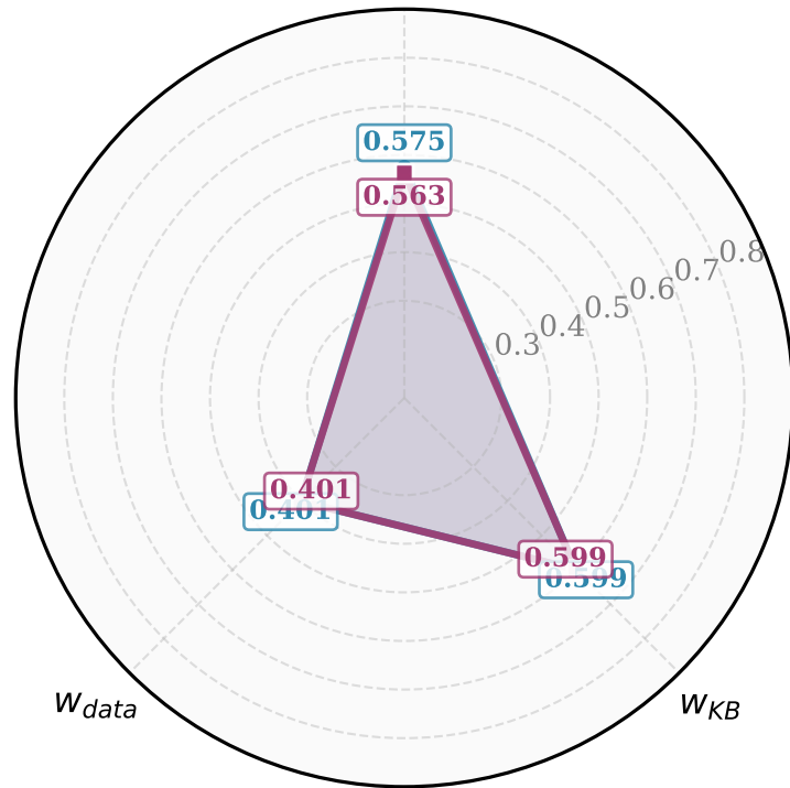
DIXIT Integrated F1
