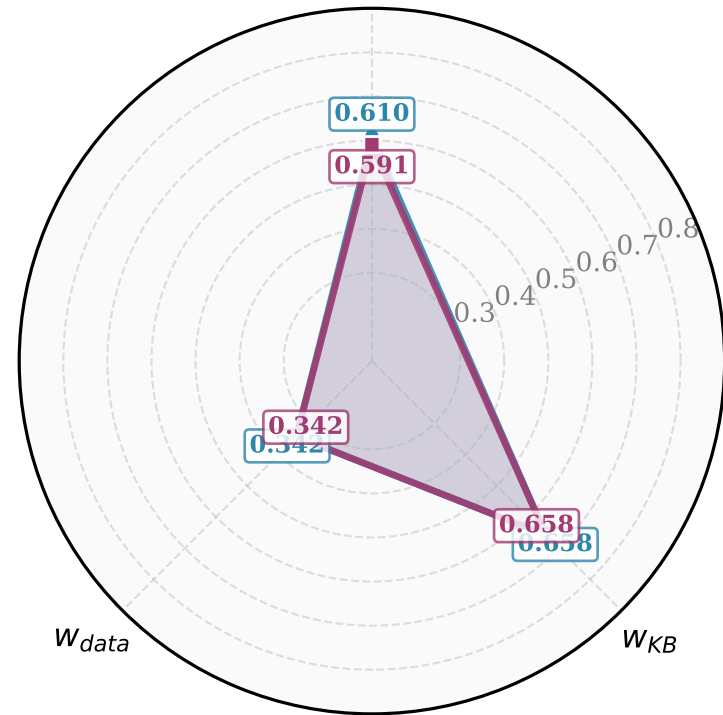
ADAMSON Integrated F1
