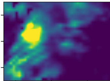
QM (3.44)
