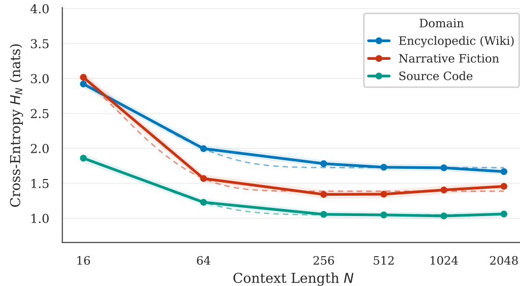
Llama-2-7b
