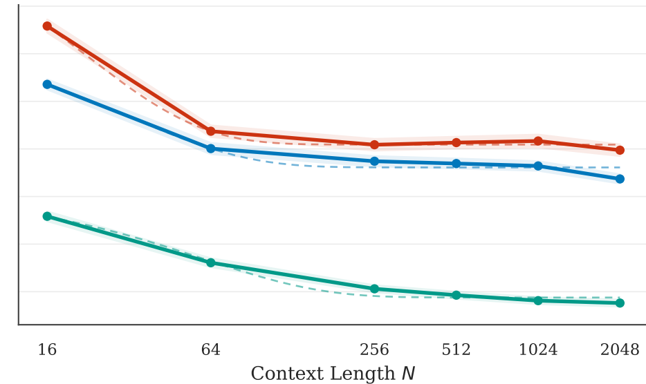
Qwen3-8B
