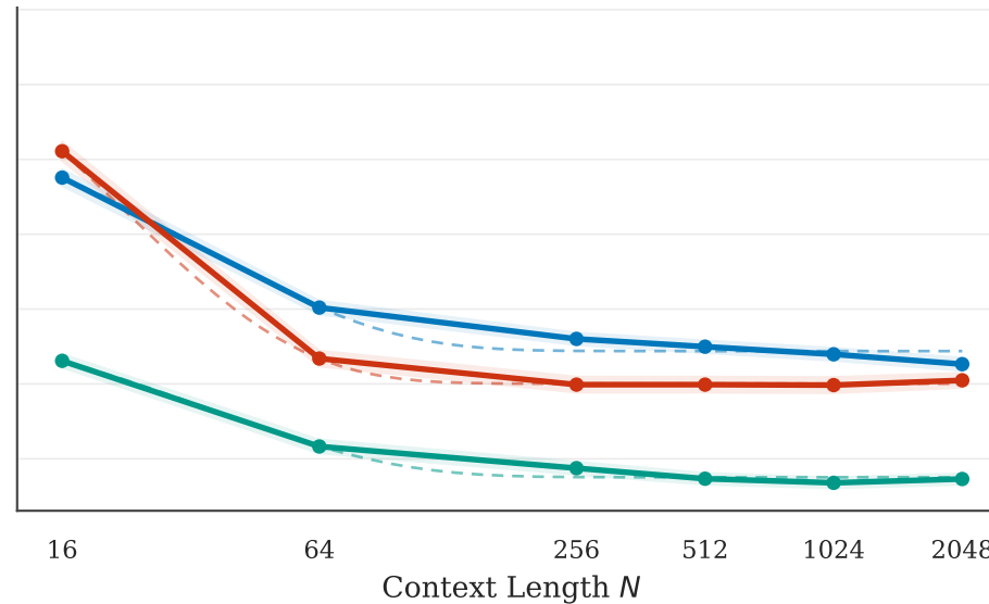
Mistral-7B-v0.1
