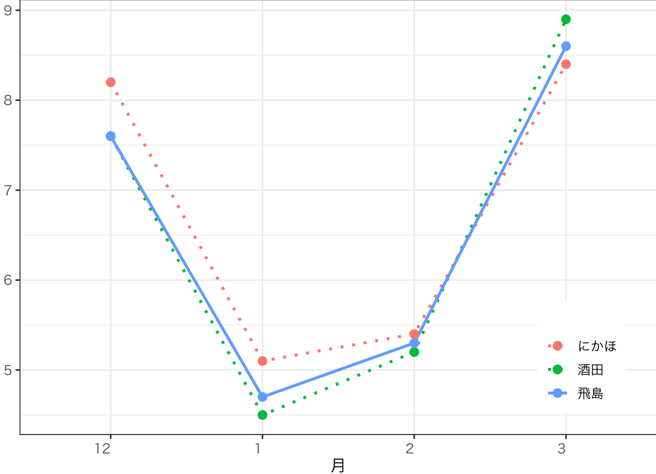
日最高气温(12月~3月) 平年値(°C)
