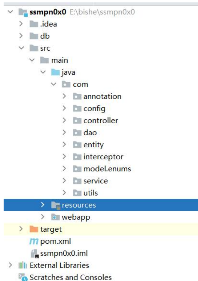
图 4.1 项目结构图
