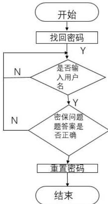
图 3.6 找回密码流程图
