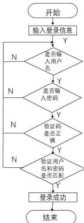
图 3.5 登录流程图
