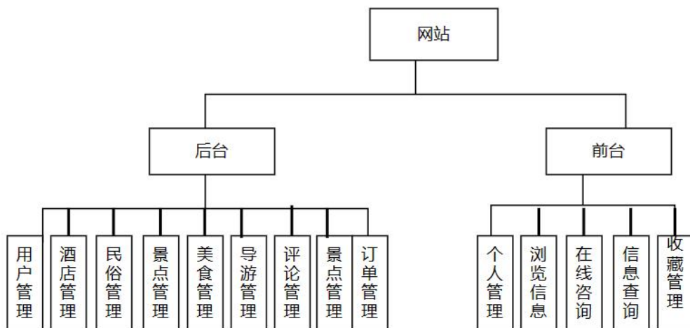
图 3.1 功能结构图
