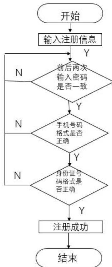
图 3.4 注册流程图
