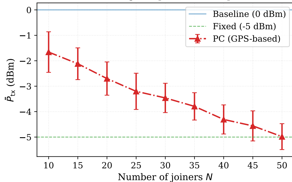
(d) Average TX power (PC adapts)
