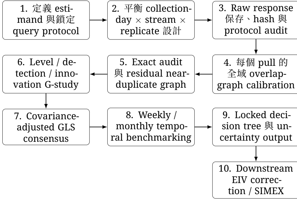
Figure 1: RACER-GT 的完整估計鏈。每一層均保留輸入、輸出與稽核紀錄；非相同 pulls 不因偏離中位數而被刪除。
