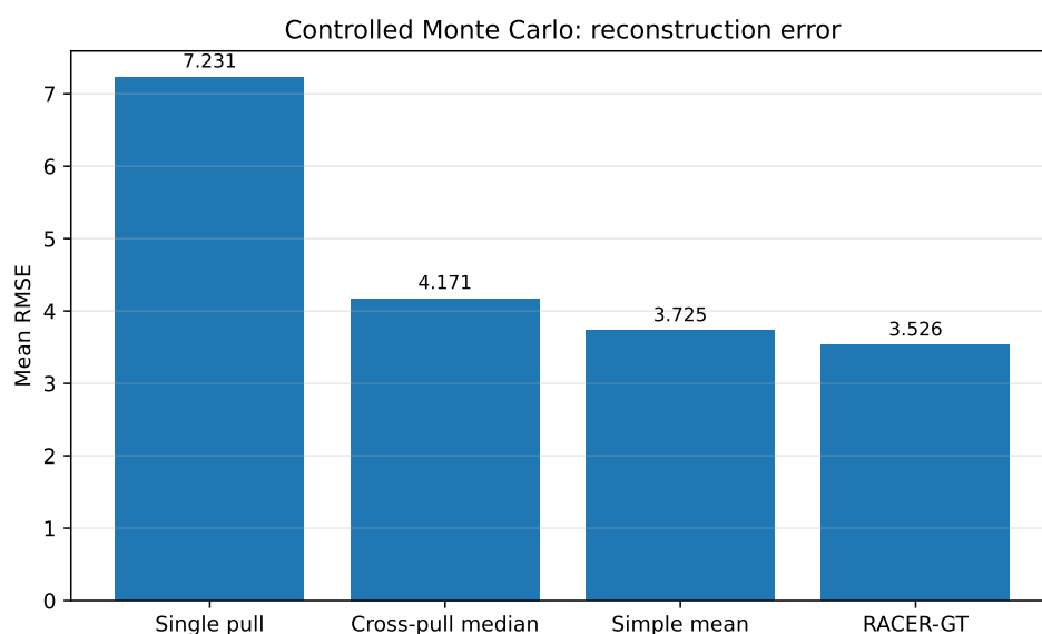
Figure 2: 不同重建方法的平均 RMSE。
