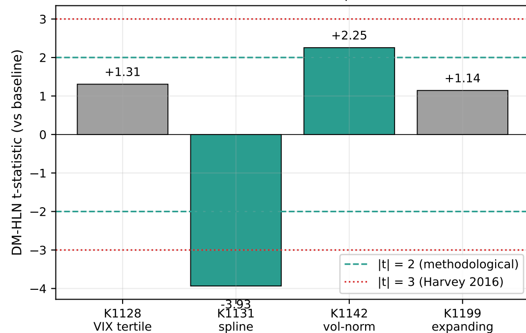
(d) Diebold-Mariano-HLN t-stat vs per-branch baseline
