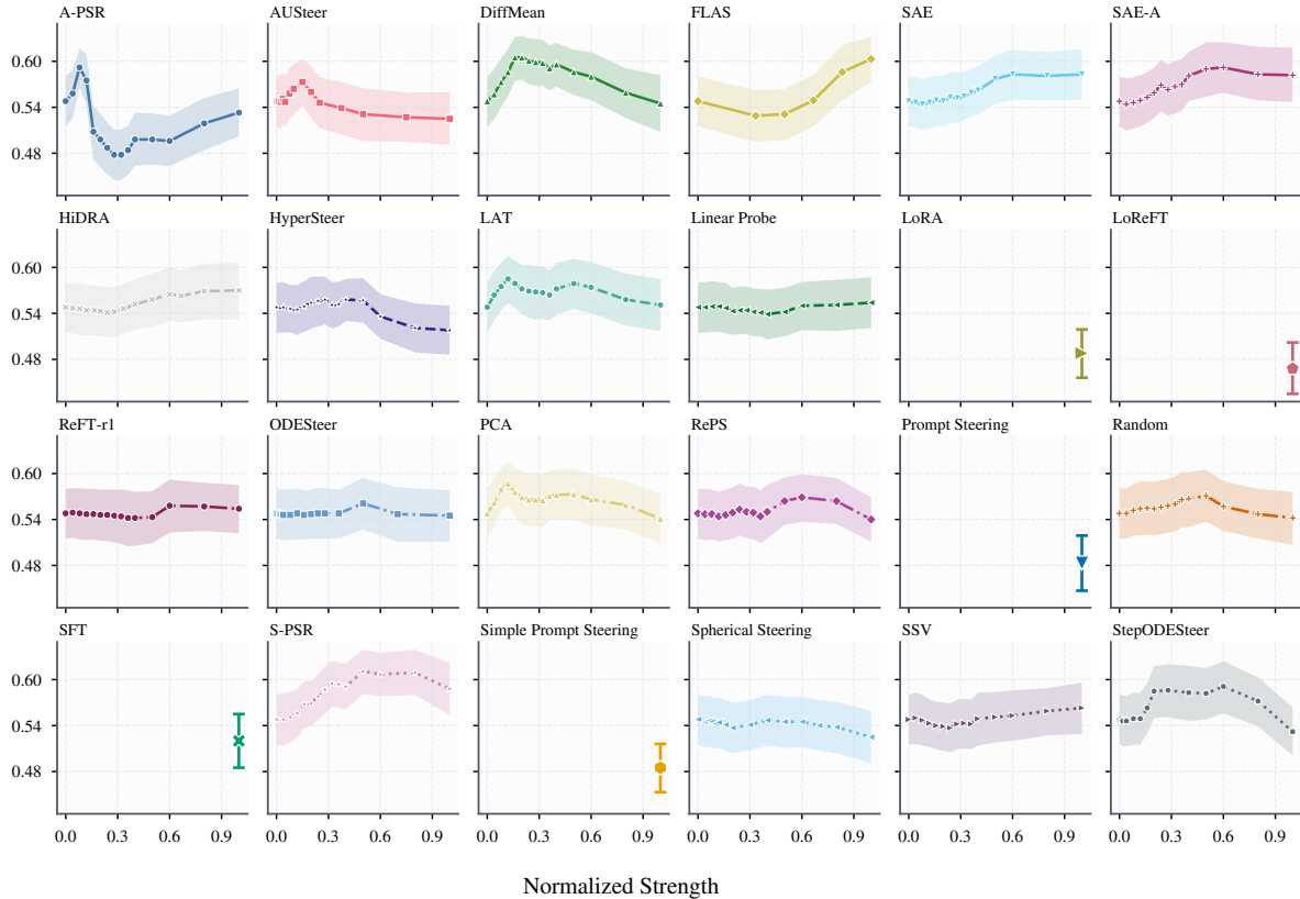
SuperGLUE W IC ↑
