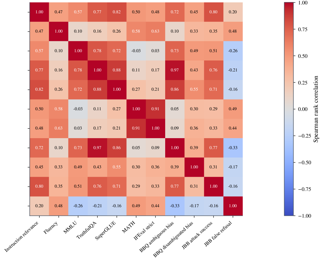
Gemma-2-9B · L20
