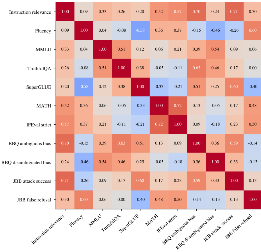
Gemma-2-2B · L20
