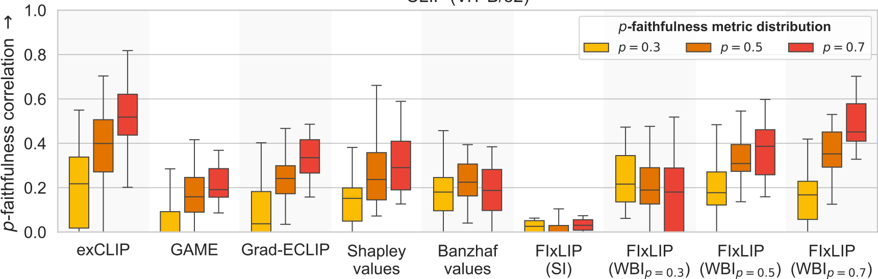
CLIP (ViT-B/32)
