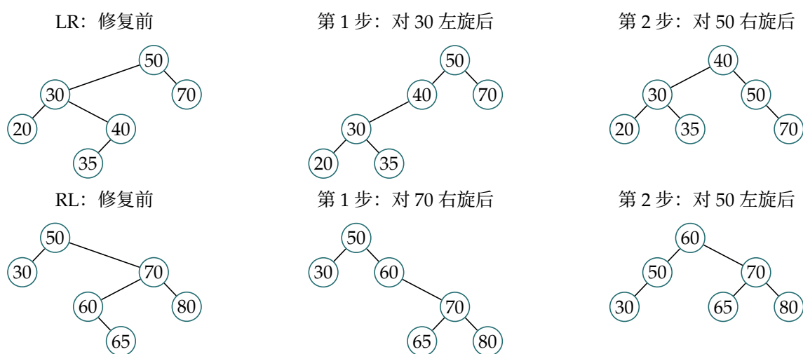
图 1.5 LR 与 RL 的双旋修复。
