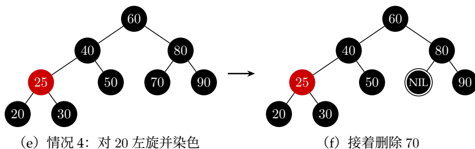
图 2.12 (e) 删除 10 并恢复平衡后的树；(f) 在此基础上删除 70，进入情况 2。
