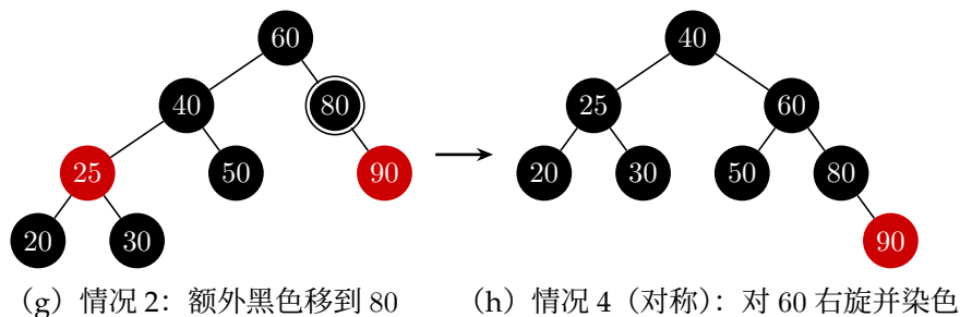
图 2.13 情况 2 把额外黑色交给 80；随后使用情况 4 的操作，完成第二次删除。
