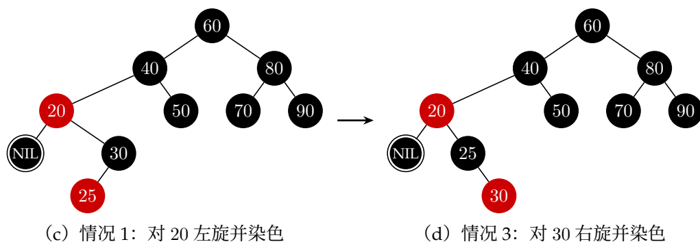
图 2.11 情况 1 之后，新兄弟满足情况 3；再次旋转后，红色结点 30 成为远侄子。
