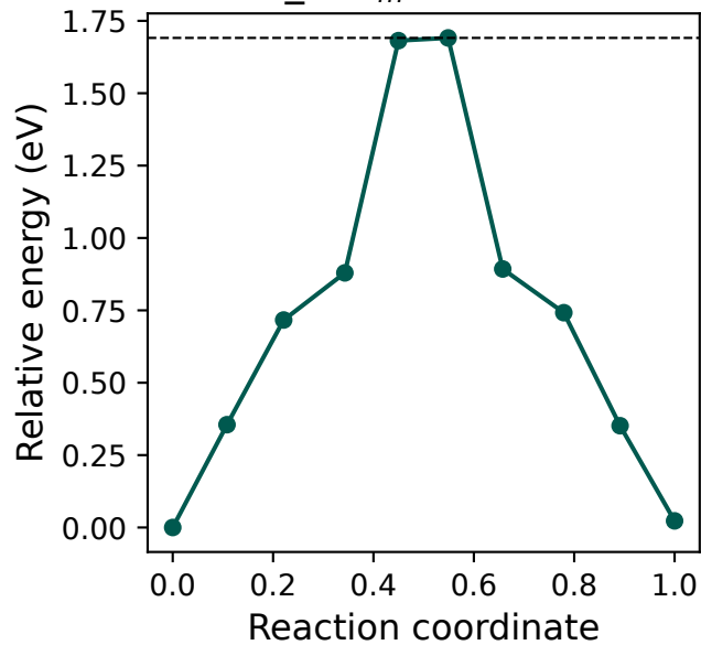
(d) neb_3: E_m = 1.691 eV
