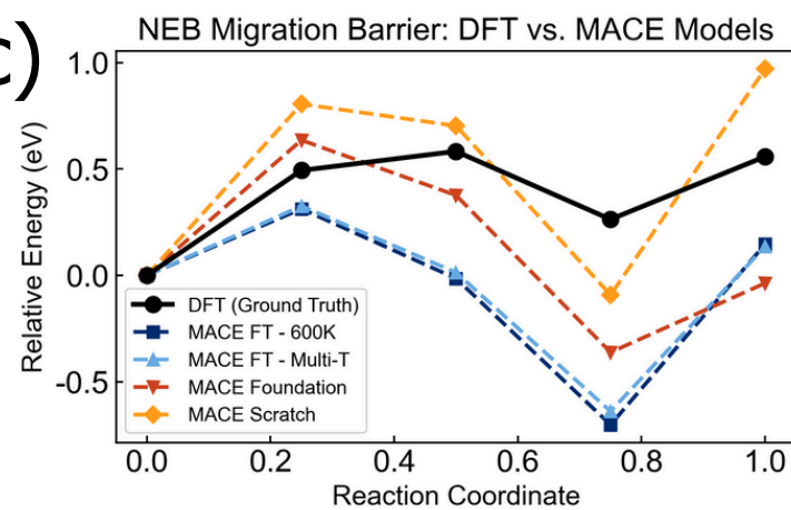
In-gap diffusion
