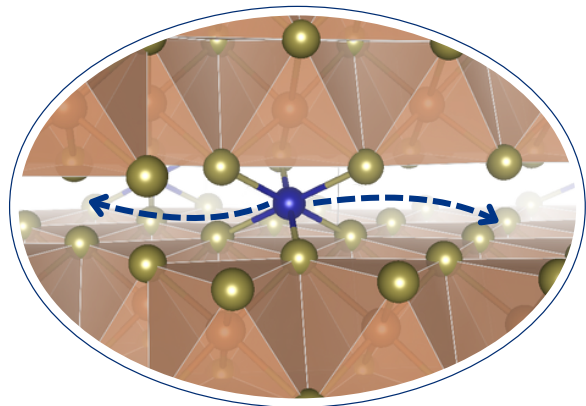
In-gap diffusion
