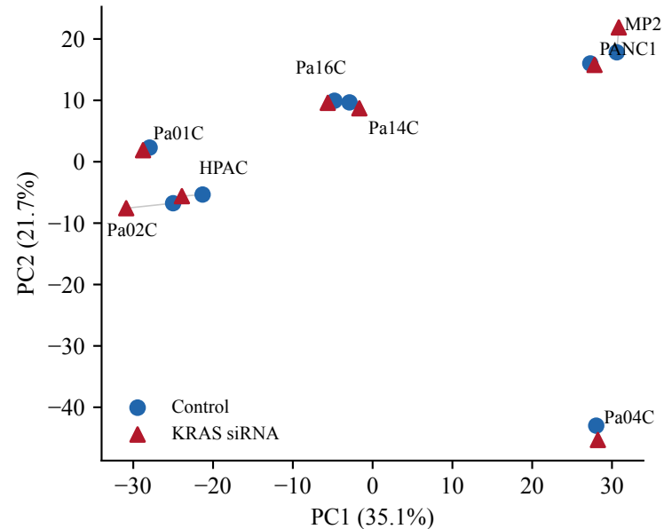
DESeq2: VST
