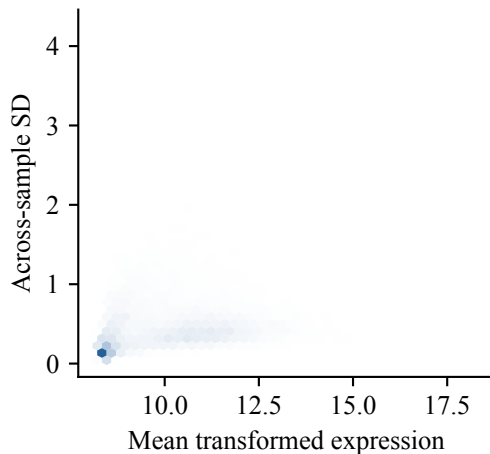
DESeq2 VST
