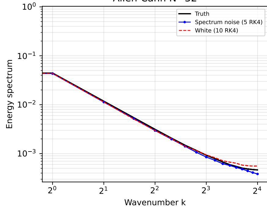
Allen-Cahn N=32
