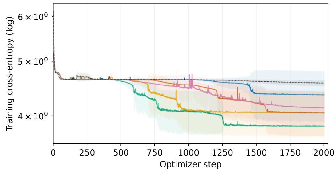
S_5 : standard
