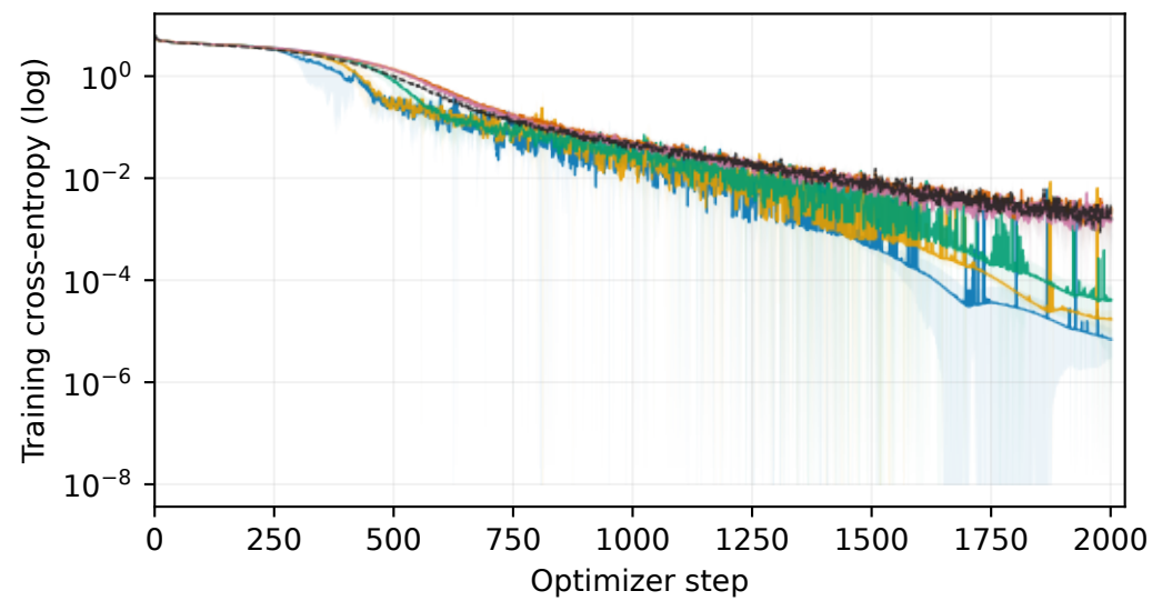
S_5 : swaps
