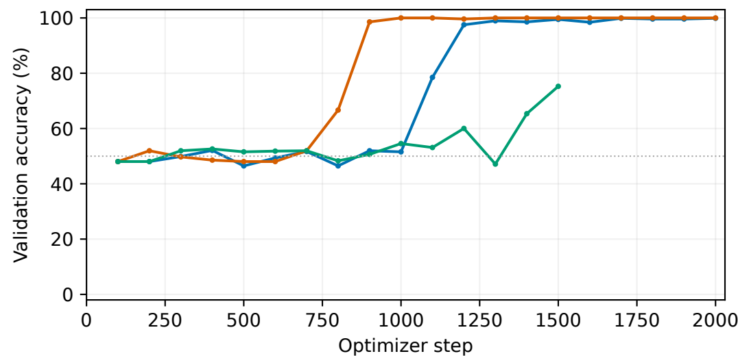
RLT 8+0
