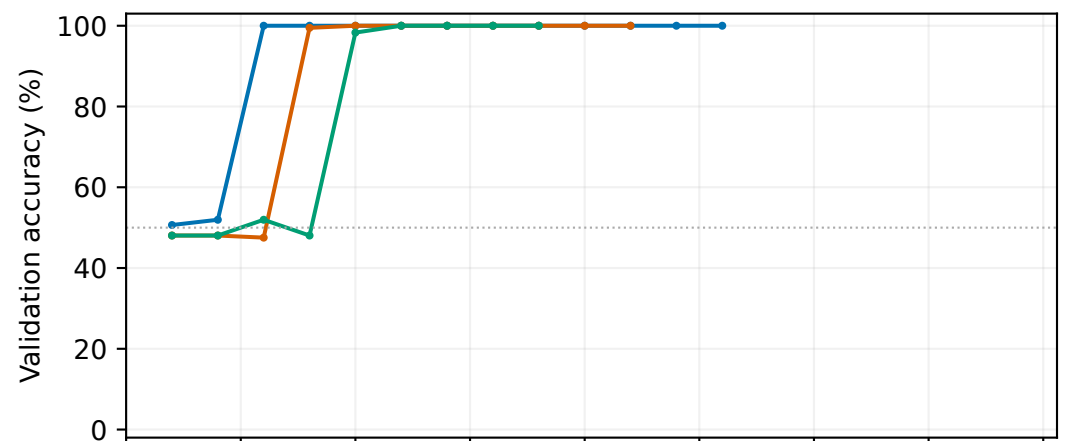
RLT 8+0
