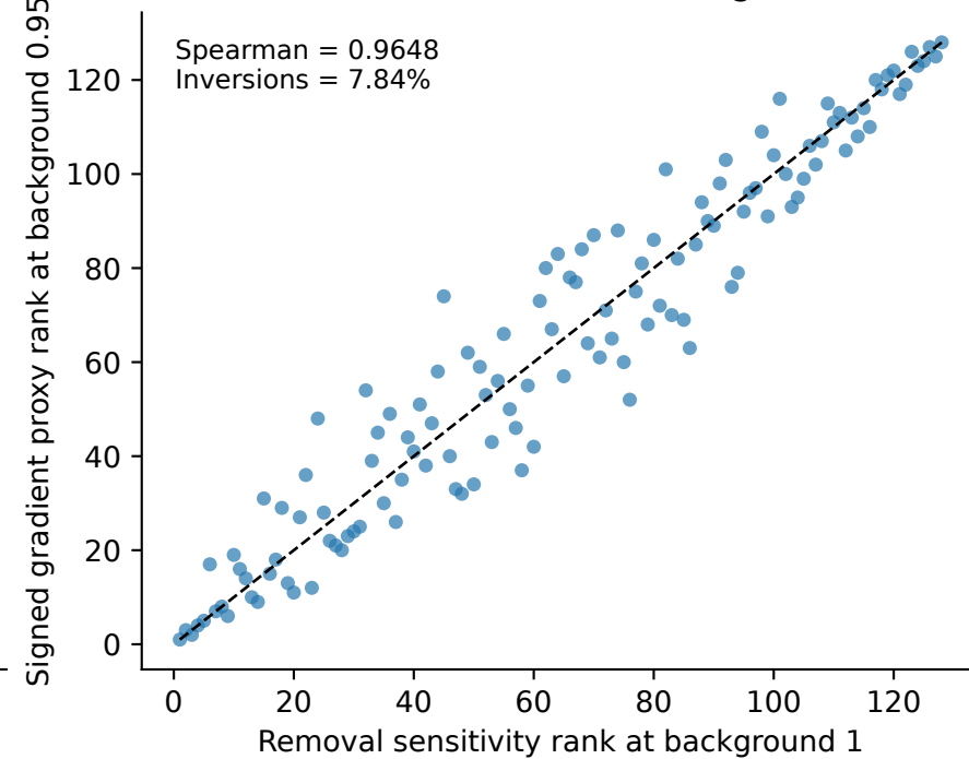
(e) Counterexample 2
