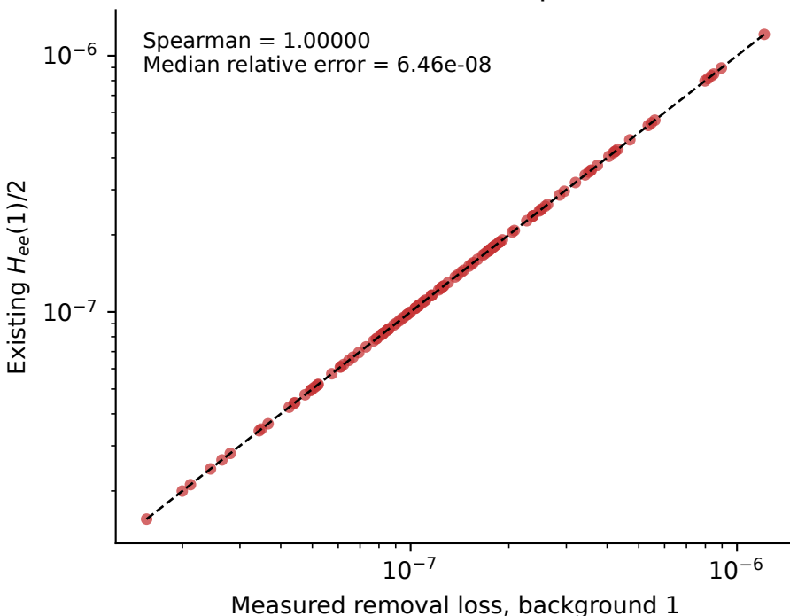
(d) Counterexample 1
