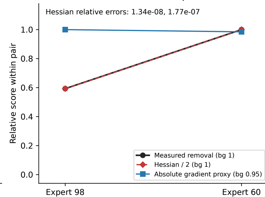
(e) Counterexample 2
