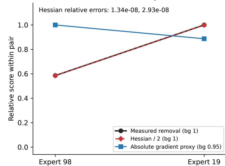
(d) Counterexample 1
