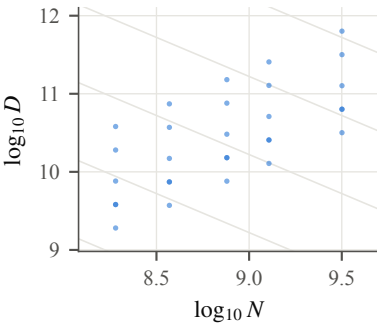
OLMo ladder: sd = 0.94
