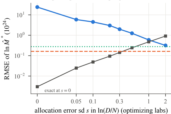
C. Compute-optimal tokens per parameter M^*
