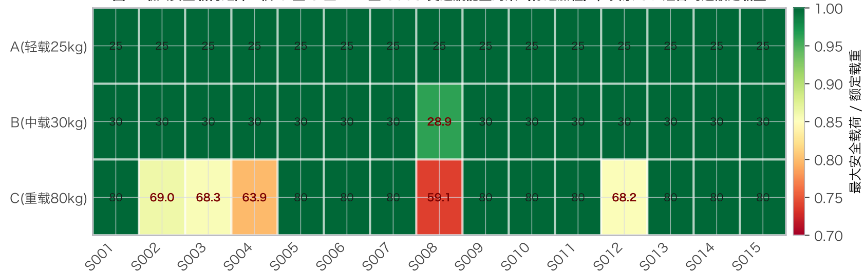
图1 最大安全载荷矩阵：仅 C 型 5 区 + B 型 S008 受返航能量约束（标红加粗），其余 39 组合均达额定载重
