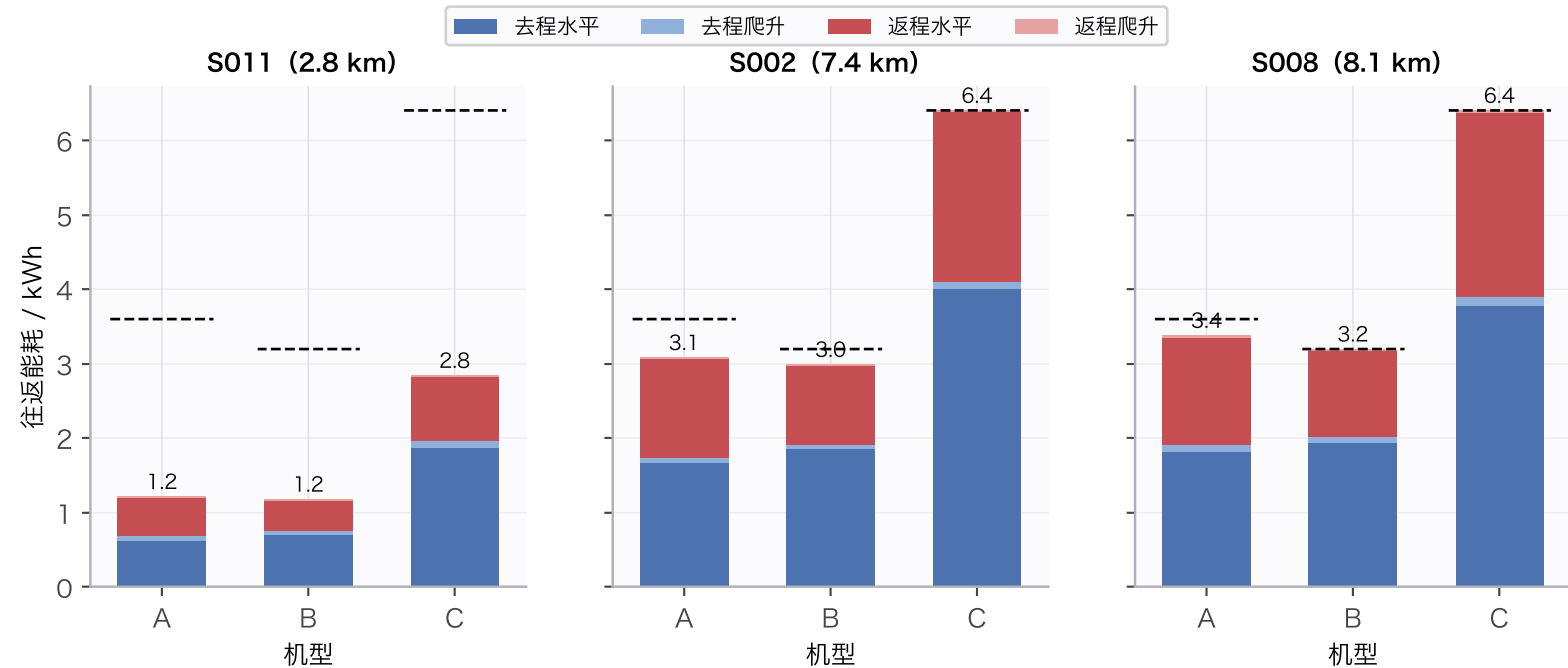
图2 单架次往返能耗分解：水平巡航能耗占主导，虚线为各机型可用能量安全上限 (1-\rho)E_{\text{use}}
