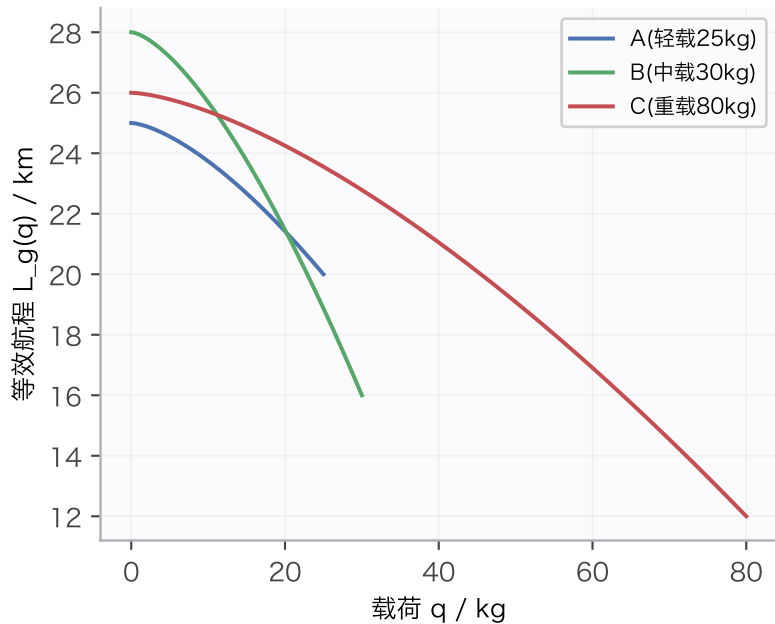
(a) 载荷 - 等效航程曲线（凹减，满载最短）
