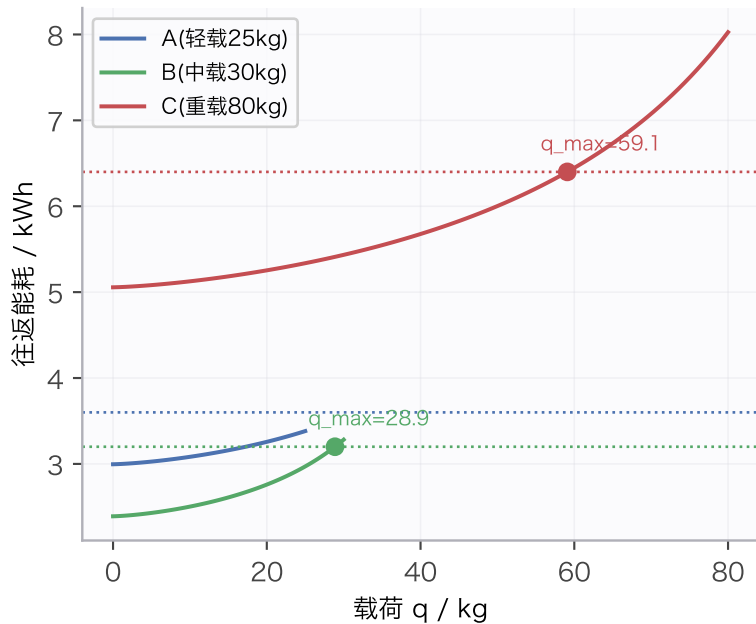
(b) S008 往返能耗随载荷单调增（点线为安全上限）
