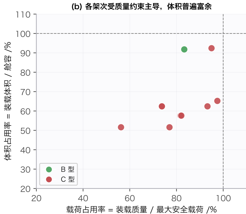
图6 货箱组批方案：18 架次(9C+9B)可行，能力瓶颈是安全载荷而非舱容
