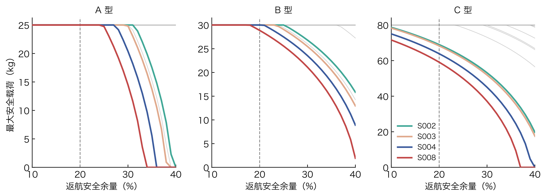
图 4.3 返航安全余量对最大安全载荷的影响
