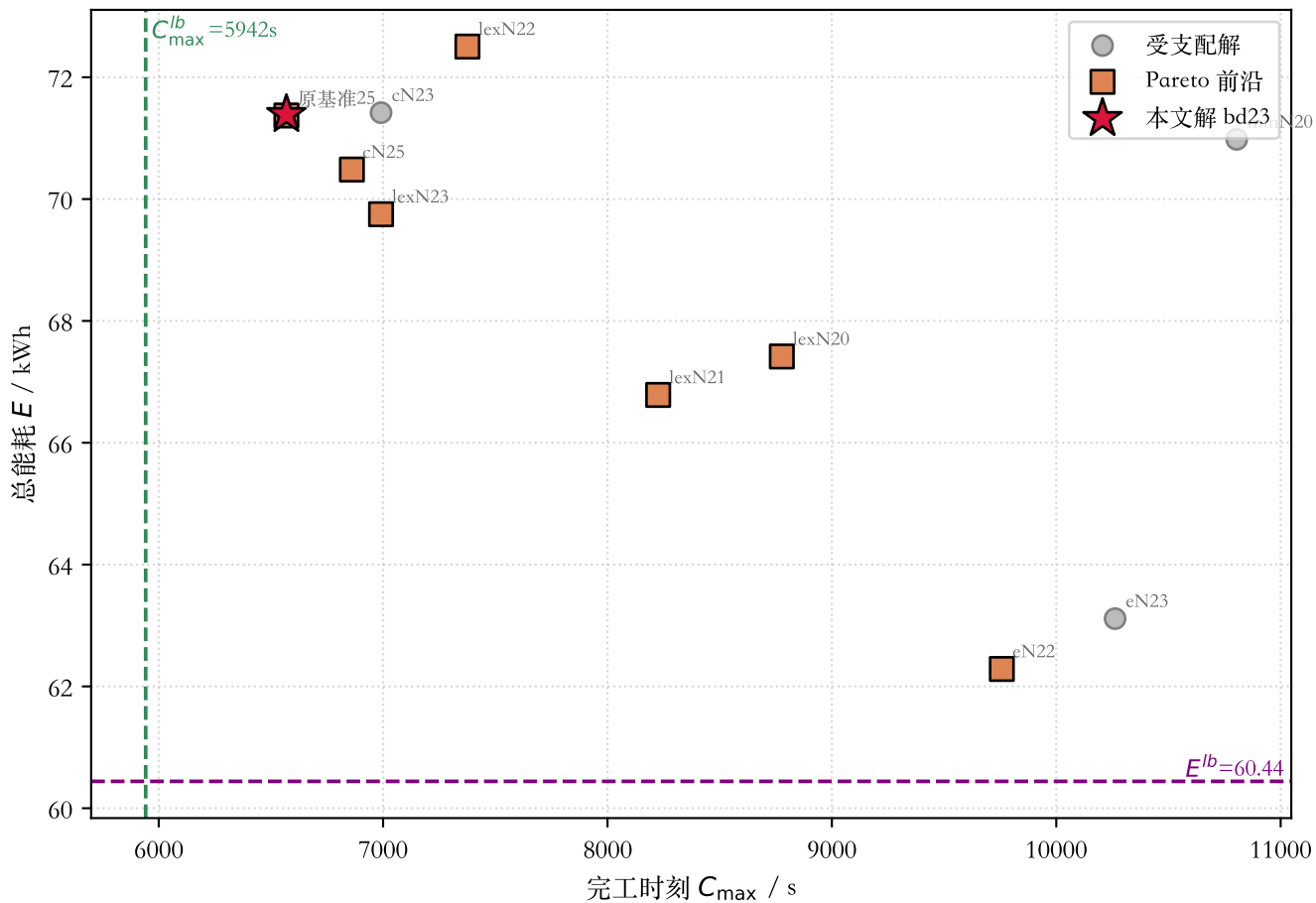
问题2 解集的 C_{\max} -能耗权衡与理论下界
