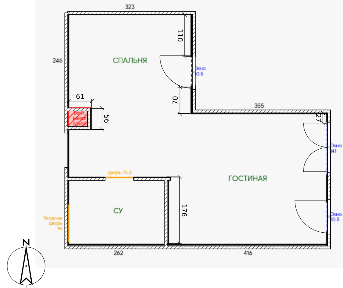
Обновленный план-подложка с вент.каналом (в см)
