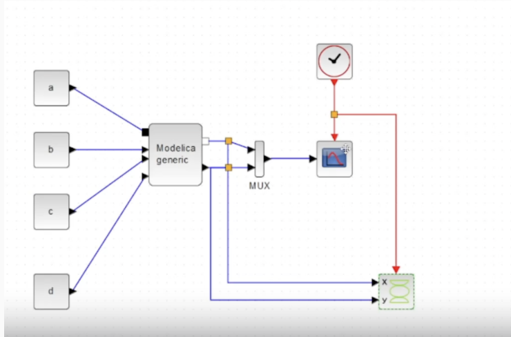
Рис. 7: Модель «хищник-жертва» в xcos с применением блока Modelica
