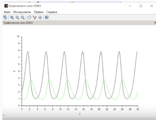
Рис. 10: Динамика изменения численности хищников и жертв модели Лотки-Вольтерры при a = 2, b = 1, c = 0.3, d = 1, x(0) = 2, y(0) = 1
