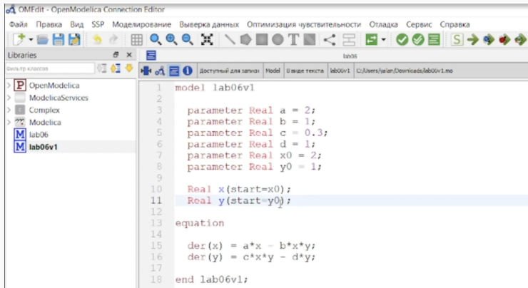
Рис. 12: Код программы
