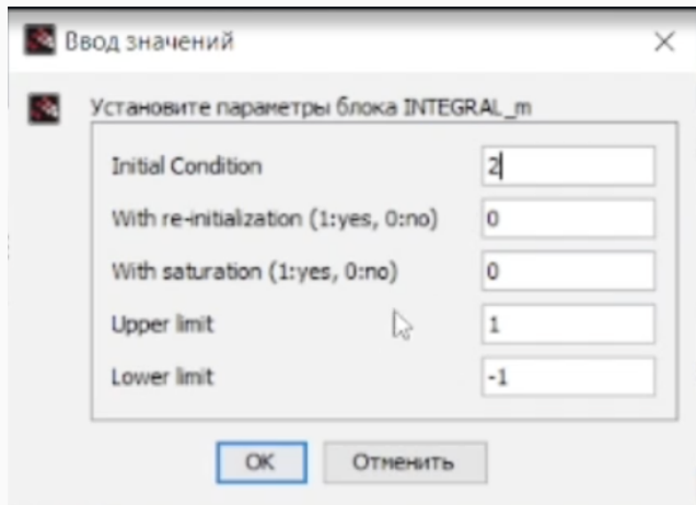
Рис. 3: Задание начальных значений в блоках интегрирования
