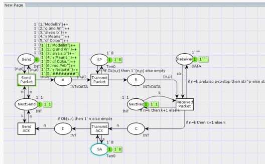
Рис. 5: Модель простого протокола передачи данных
