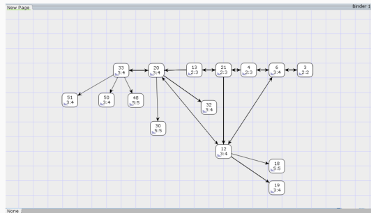
Рис. 7: Пространство состояний для модели простого протокола передачи данных
