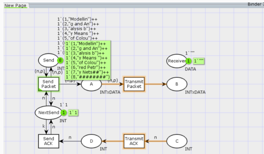
Рис. 3: Добавление промежуточных состояний
