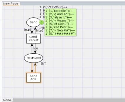
Рис. 2: Начальный граф
