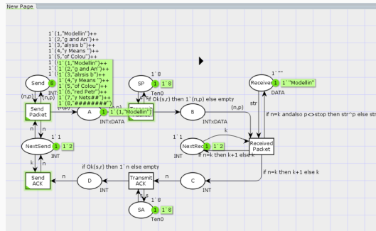
Рис. 6: Запуск модели простого протокола передачи данных
