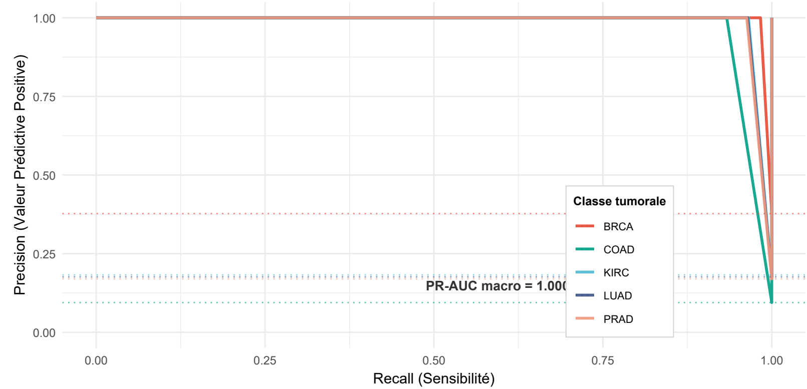
b (b) Courbes Precision-Recall par classe Lignes pointillées = baseline (prévalence de la classe)
