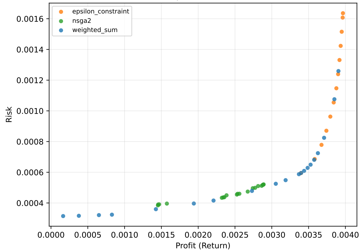
port5 (K=8)
