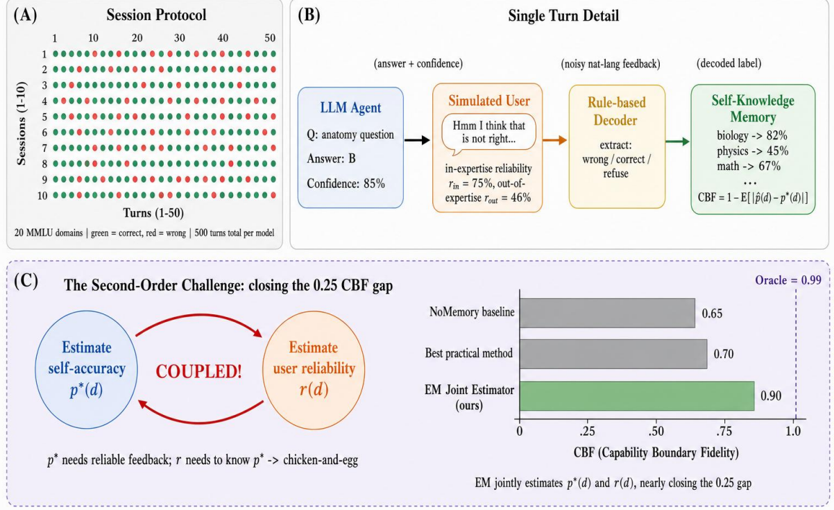
图 1: SelfBound 概览: H3 是核心挑战。(A) 会话协议: 每会话 50 轮, 问题从 20 个 MMLU 领域中抽取 (绿色 = 正确、红色 = 错误)。(B) 单轮: 智能体带置信度作答, 跨家族模拟用户给出域依赖的噪声反馈 (域内 r_{in} \approx 75\% 、域外 r_{out} \approx 46\% ), 解码器提取标签信号, 按领域更新自我模型; CBF 衡量 \hat{p} 与真实 p^*(d) 的逐域保真度。(C) H3 的核心挑战: 智能体必须同时估计自身分领域准确率 p^*(d) 与模拟用户可靠性 r(d) ——两者耦合 (要估 p^* 需要可靠反馈、要估 r 需要知道 p^* , 鸡生蛋问题)。EM-Joint 等二阶联合估计器能闭合该 0.25 CBF gap 中的大部分 (详见 §5)。
