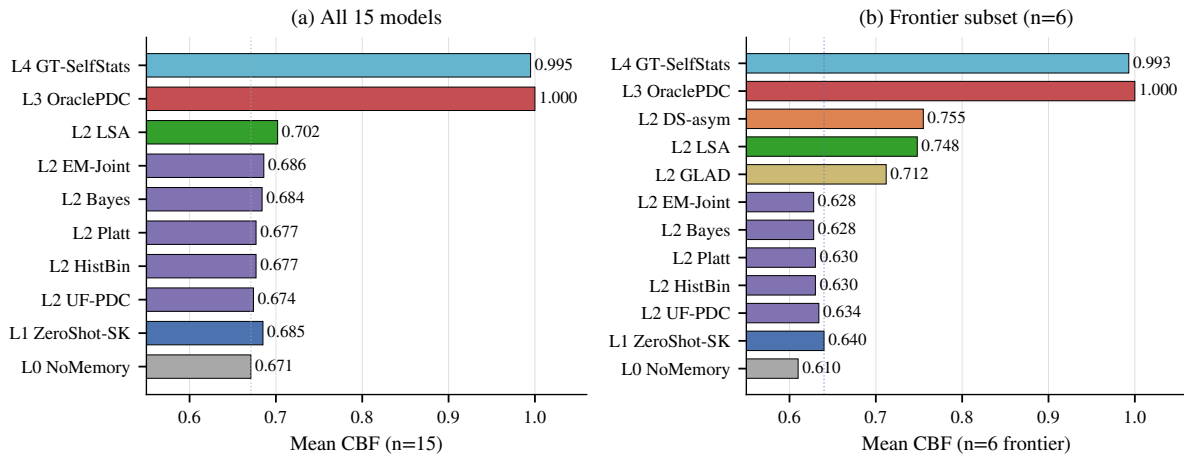
图 2: 五级诊断阶梯。每个基线级别的平均 CBF: (a) 所有 15 个模型; (b) 6 个前沿模型。(a) L2→L3 差距约 0.30 (最佳 L2 LSA 0.702 vs. OraclePDC 1.000): 一阶 L2 方法无法从噪声反馈中恢复信号。(b) 在前沿子集上, 一阶 L2 集群 (Platt/HistBin/Bayes/EM/UF) 坍塌至 NoMem (0.628–0.634), 而二阶估计器 (DS-asym 0.755、GLAD 0.712) 和上下文 LSA (0.748) 干净地超过 L1 ZS 先验 (0.640)。垂直点线标记 L0 NoMemory 锚点。
