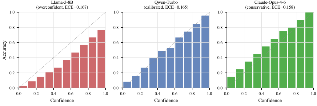
图 5: 三种可靠性特征。三个代表性智能体的每 bin 准确率 vs. 置信度, 展示了典型模式: Llama-3-8B (过度自信: 柱条低于对角线)、Qwen-Turbo (校准良好: 柱条沿对角线)、Claude-Opus-4-6 (保守: 柱条高于对角线)。每 bin 值由每模型整体 ECE (表 2) 重构; 定性形状为经验, 每 bin 粒度为示意。
