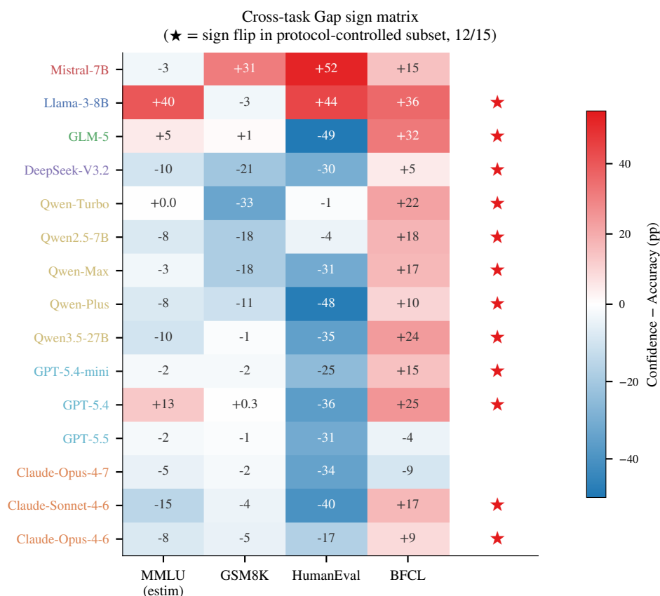
图 9: 跨任务 Gap 符号矩阵。每个单元显示 MMLU/GSM8K/HumanEval/BFCL 的每模型置信度-准确率 Gap (pp); 红色 = 过度自信, 蓝色 = 保守。右侧 ★ 标记在三个同协议扩展任务上至少出现一次符号反转的模型 (12/15 = 80%)。MMLU 列由每模型 NoMem-准确率比较估计而来, 仅作参考显示; 符号反转计数仅使用三个同协议任务。
