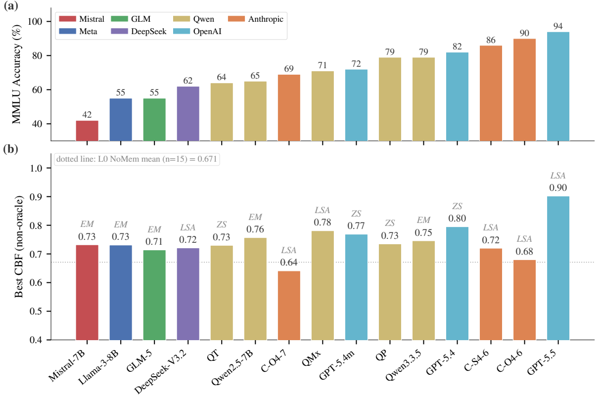
图 3: 15 个模型的能力谱。(a) MMLU 准确率从 42% 到 94%; 家族颜色在全文中保持一致。(b) 每个模型的最佳非预言机 CBF 及获胜基线标签 (EM/LSA/ZS)。点线标记 L0 NoMemory 均值 ( n=15 , 0.671)。两个新增的前沿模型 (GPT-5.5、Claude-Opus-4-7) 锚定了高准确率端。注意 Claude-Opus-4-7 的 MMLU 准确率较低 (69%), 但被纳入 n=6 前沿子集用于二阶分析。
