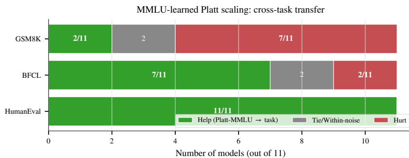
图 10: MMLU 学习的 Platt 缩放：跨任务迁移 。在每个目标任务上，迁移后的重新校准对模型（11 个有可用 MMLU Platt 参数）有帮助、打平或有害的数量。在 HumanEval 上有帮助（11/11），但在 GSM8K 上有害（7/11），证实了从 MMLU 典型过度自信学到的”置信度收缩”会损害已经保守的 GSM8K 模型——每任务边界是结构性必要而非便利。
