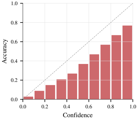
Llama-3-8B (overconfident, ECE=0.167)
