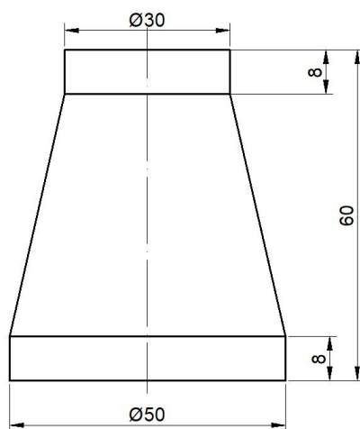
图 5 决赛第一阶段的物料形状
