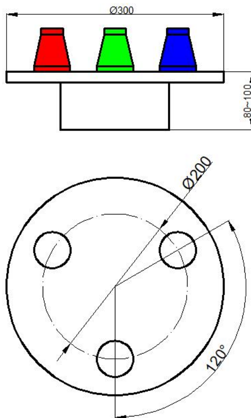
图 2 原料区示意图（颜色仅供参考）
