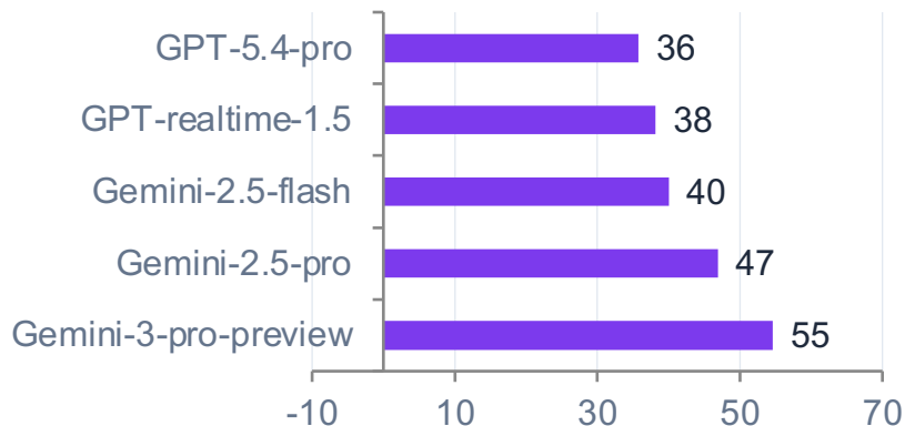
AudioMultiChallenge (Text Output)
